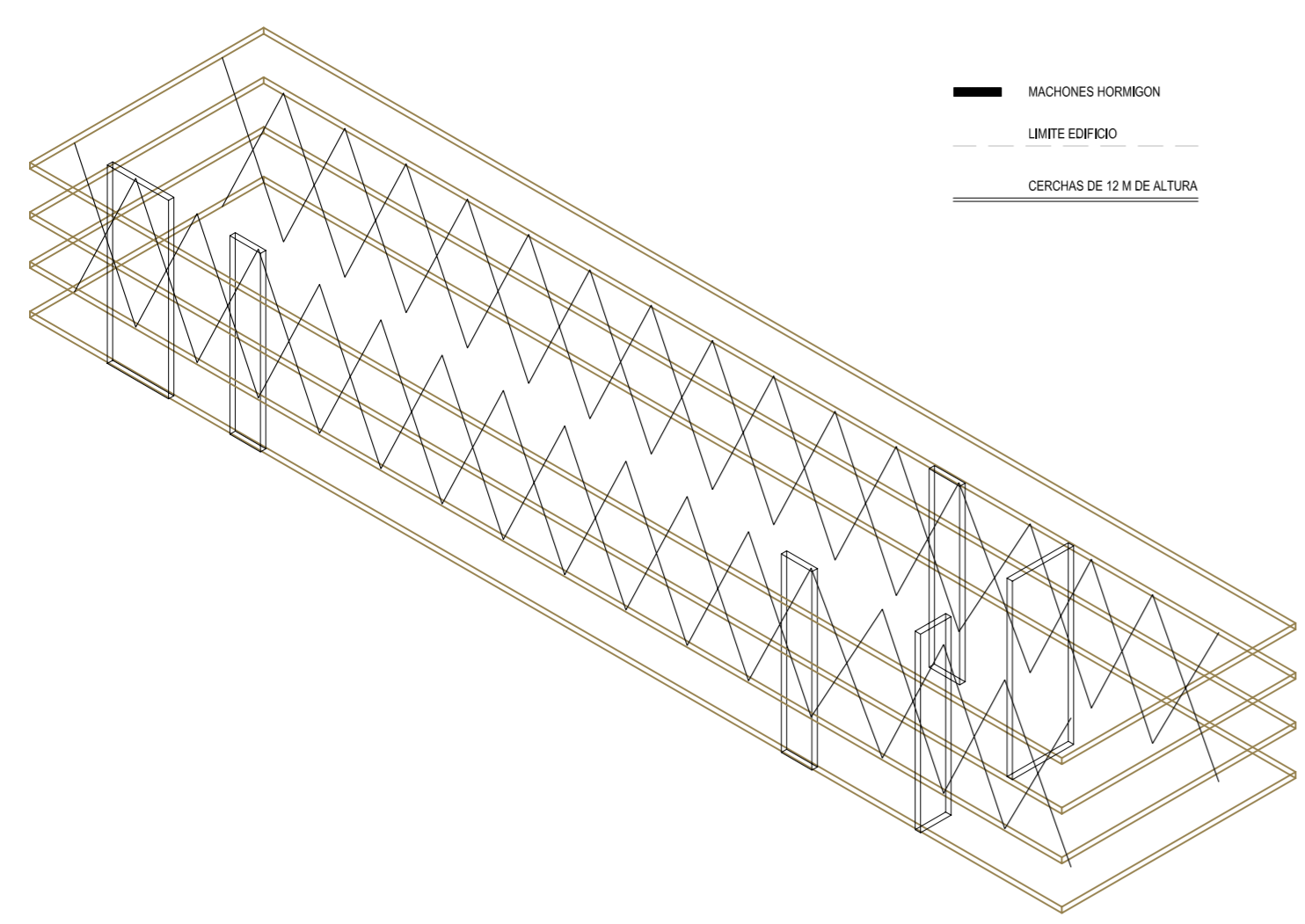
ESQUEMA ESTRUCTURAL
